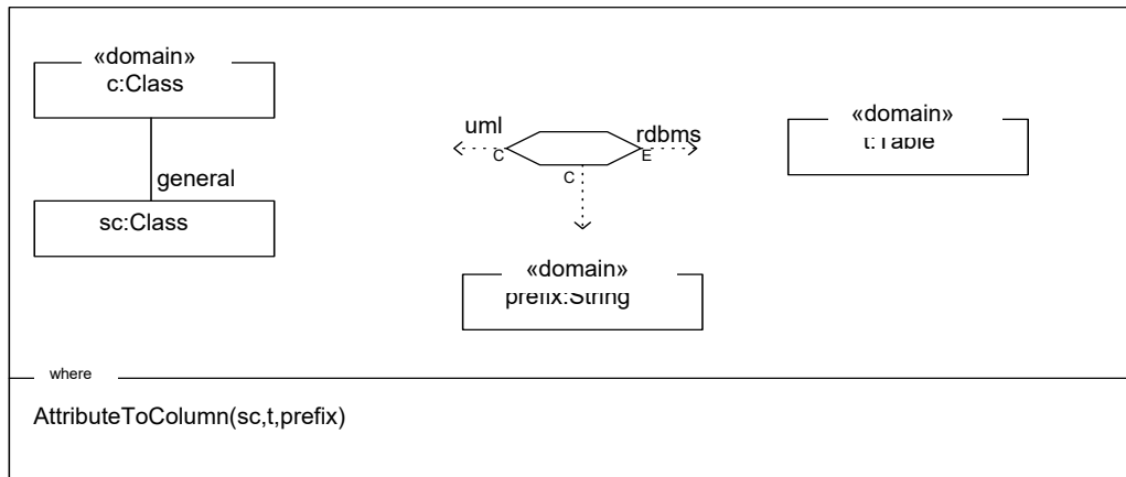
SuperAttributeToColumn
